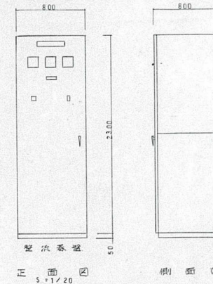
図 3 外形図
