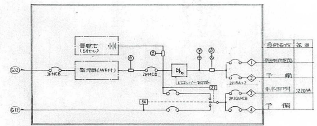
直流電源装置 結線図
