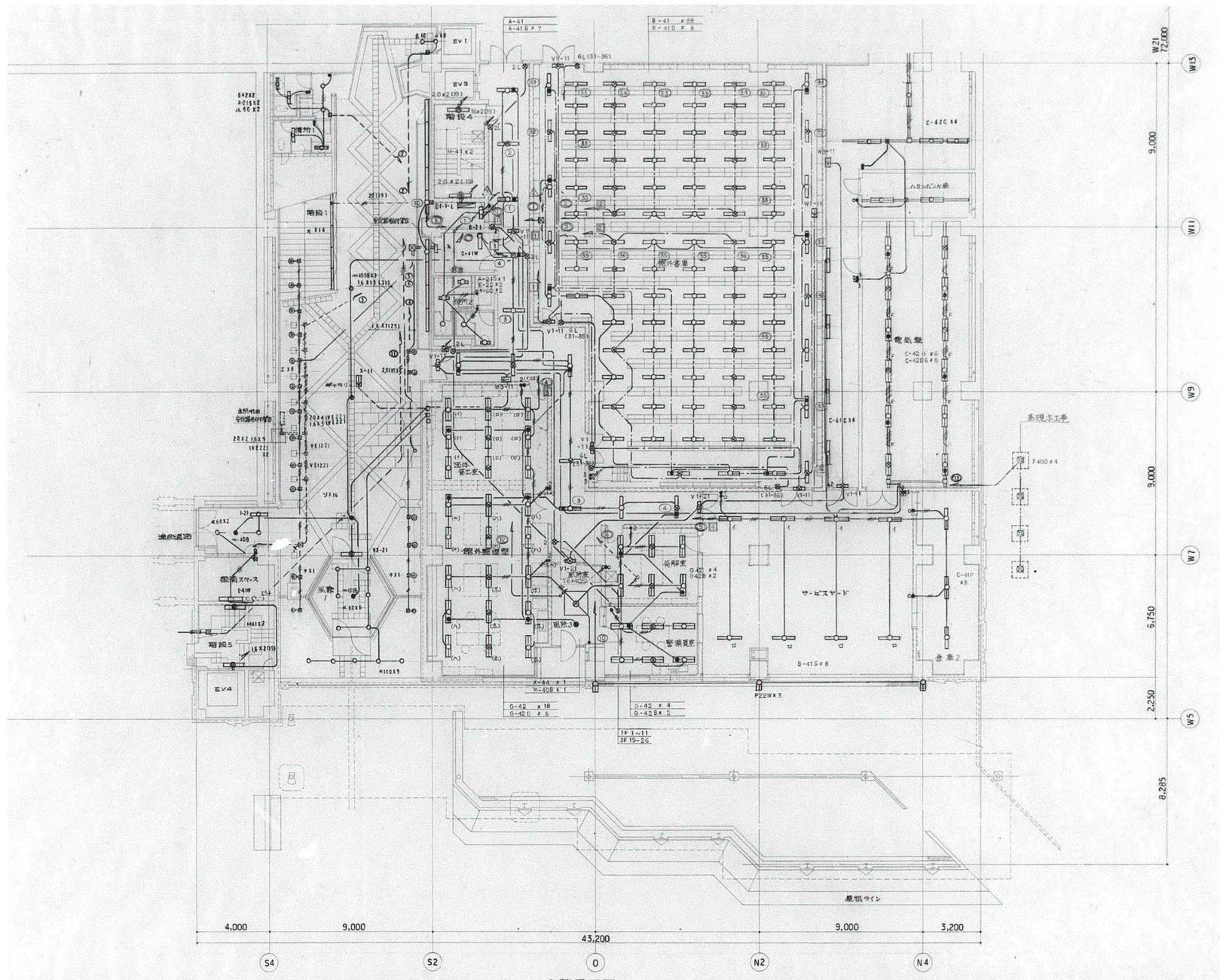
(図書館 電灯設備図 (代表階))
